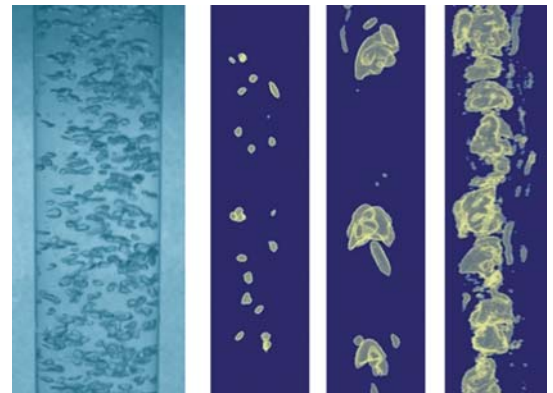
Visualisierung von aufsteigenden Gasblasen in einer Blasensäule. Links mit einer Hochgeschwindigkeitsvideokamera, rechts dreidimensionale Bilder der ultraschnellen Elektronenstrahl-Tomographie.
