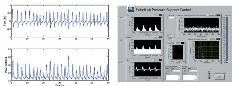
Links: typische Verläufe von Flow und Atemwegsdruck (Paw) unter assistierter Spontanatmung mit noisy pressure support ventilation (noisy PSV) an einem tierexperimentellen Modell des acute respiratory distress syndrome (ARDS); Rechts: Bedienungsfläche der noisy PSV Steuerungssoftware. (Foto: Prof. Dr. Marcelo Gama de Abreu, Dr. Alexander Krüger)
