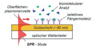
Abb. 2: Oberflächenplasmonenresonanz zum Nachweis biomolekulare Analyten mittels selektiver Fängermoleküle
