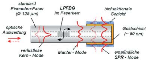
Abbildung 1: Schematische Darstellung des Sensorskonzepts.
