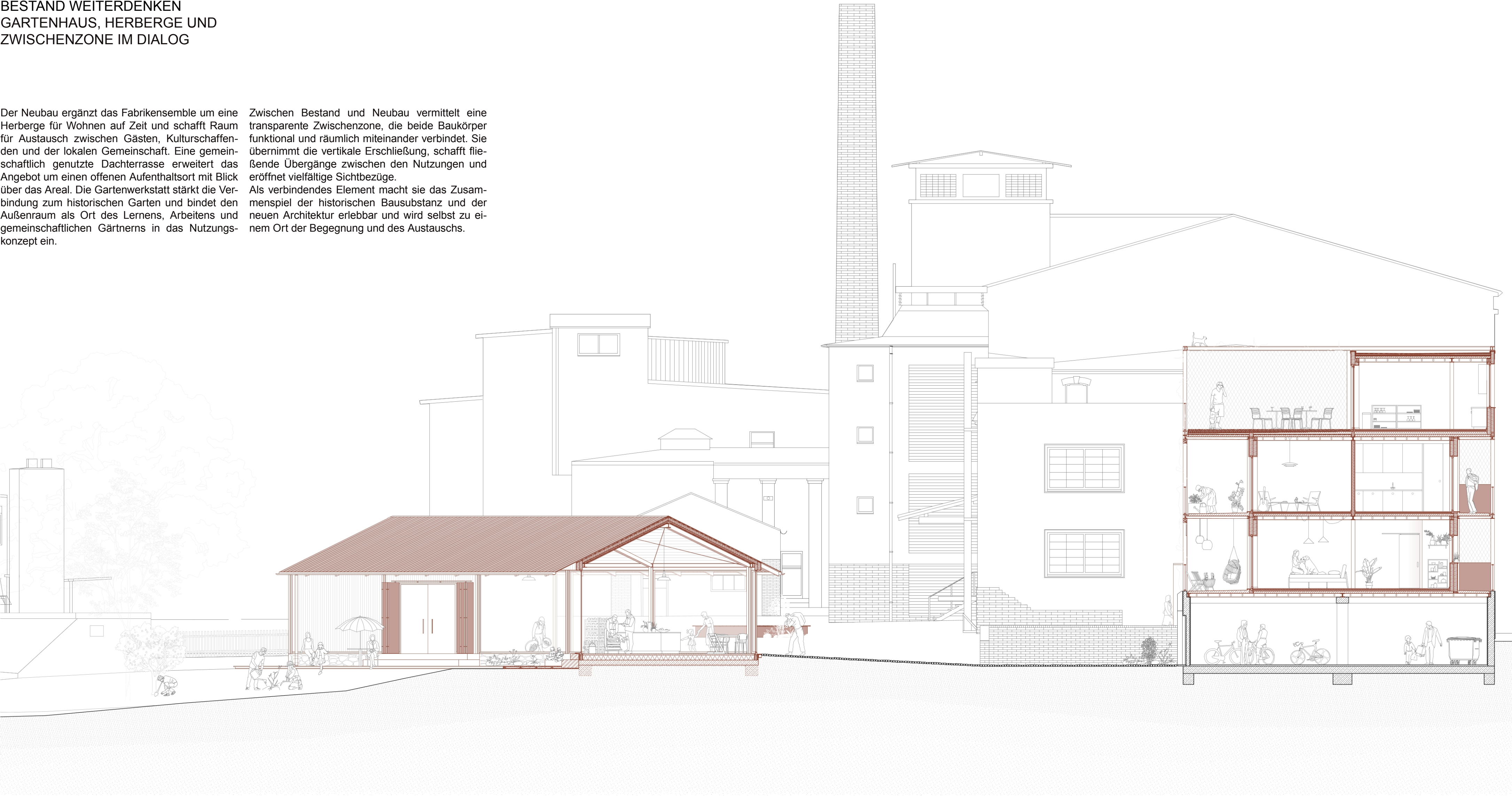
Fassadenschnitt vom Hof in Zusammenhang mit Gartenhaus und Herberge
