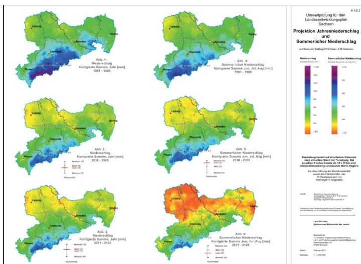
Umweltprüfung für den Landesentwicklungsplan Sachsen 2012: Projektion Jahresniederschlag und Sommerlicher Niederschlag auf Basis der Wettreg2010-Daten, A1B Szenario für die Perioden 2036 - 2065 und 2071 - 2100 sowie Vergleichsperiode 1969 - 1990.
