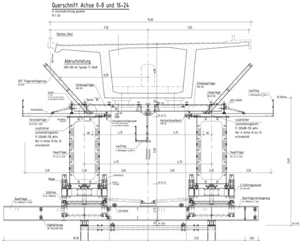
Bild 7 Brückenquerschnitt mit Abbruchwanne und Traggerüst Zeichnung: Thyssen Krupp, Wuppertal, Saul Ingenieure Braunschweig, Hörnig
