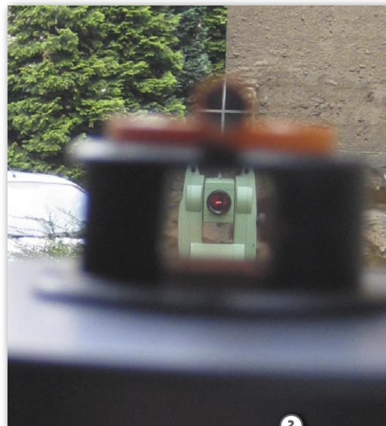
Cel w krzyżu nitek (tachimetr w przyzmacie)
