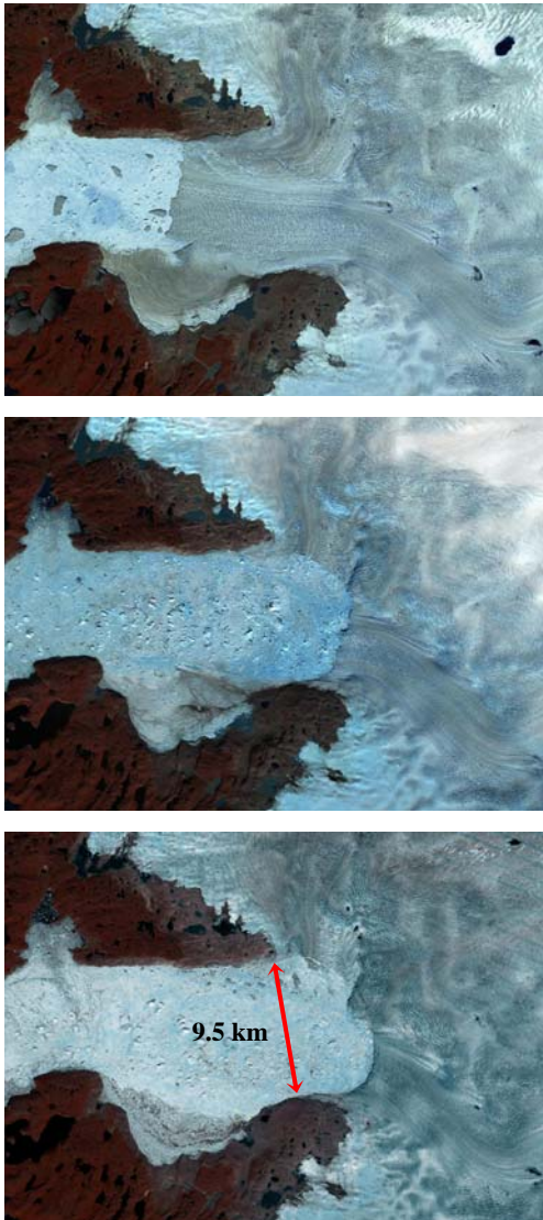
Figure 2: False color Landsat images of Jacobshavn Isbræ (7.7.2001, 8.9.2004, 8.7.2007)
