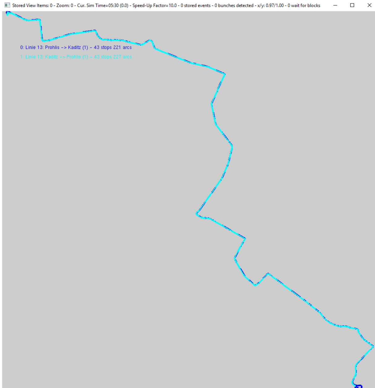
Abbildung 25: Simulationsfenster mit den beiden spezifizierten Linienverläufen der Linie 13
