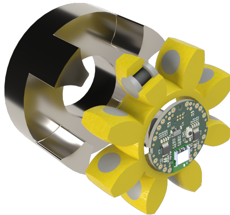
Abbildung 1: Prototyp der sensorintegrierenden Zahnkranzkupplung.
