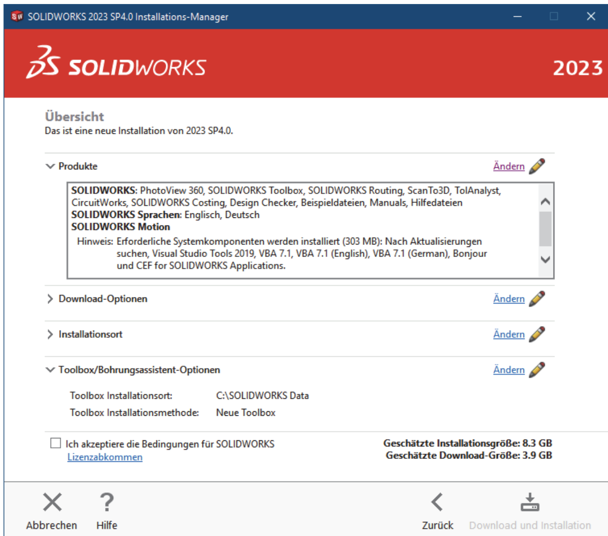
Bild 3: Übersicht
