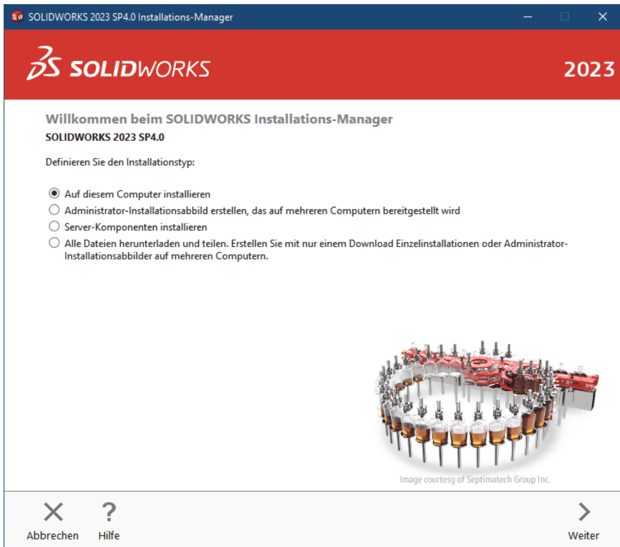
Bild 1: Willkommen
