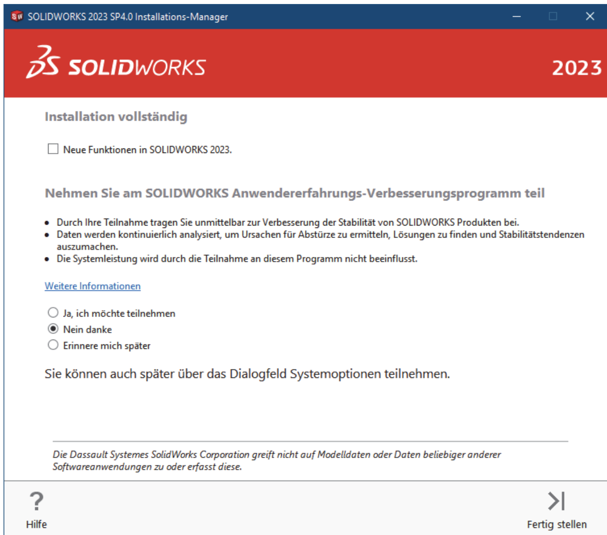
Bild 6: Installation abgeschlossen
