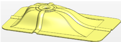
Demonstratorbauteil Federdom
