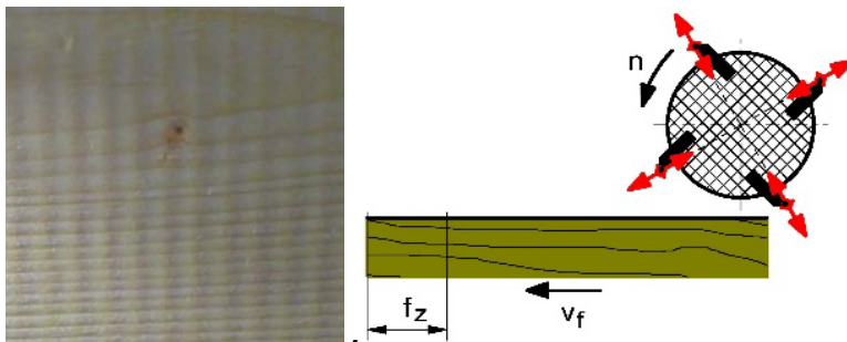
Abb. 1: links: Messerschläge auf einem Holzwerkstück; Mitte: Konzept der Messerschlagkompensation; rechts: schematische Darstellung des aktiven Werkzeugs in einer Umfangsfräsmaschine
