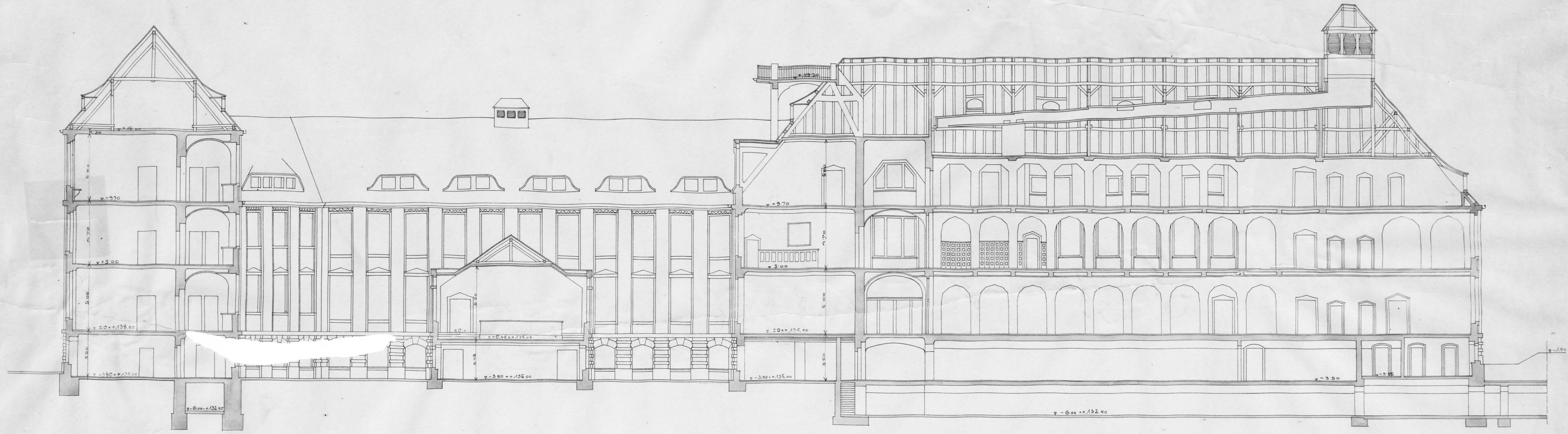
Schnitt E-F.
